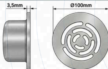
Retorno Alta Vazão 85mm
