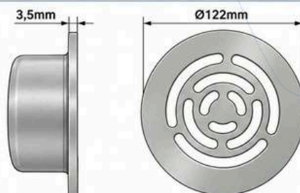
Retorno Alta Vazão 110mm
