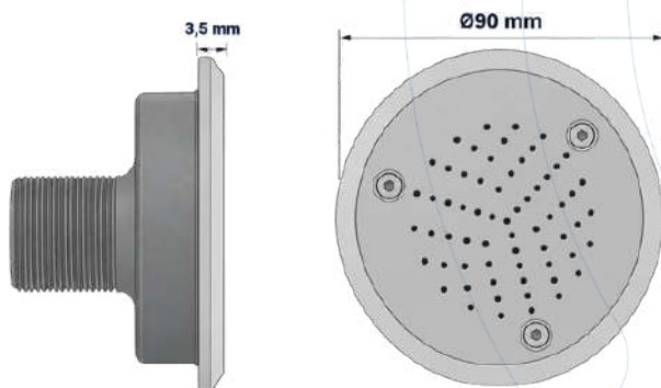
AREJADOR DE PISO ORIFÍCIOS ALINHADOS Ø90 mm
