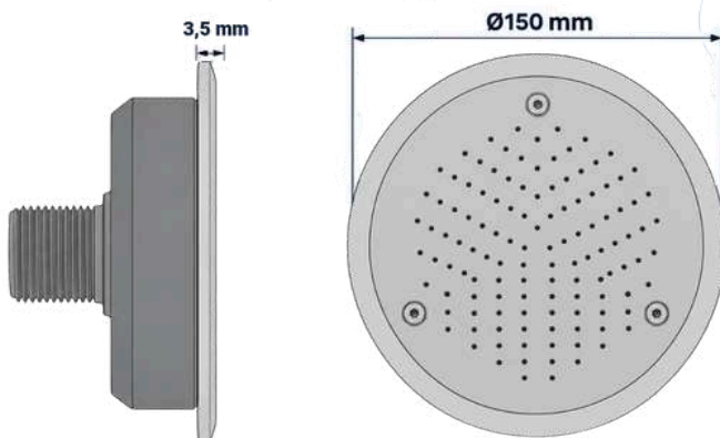
AREJADOR DE PISO ORIFÍCIOS ALINHADOS Ø150 mm
