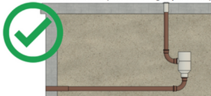
Canhão na Vertical (entrada de água para cima)
